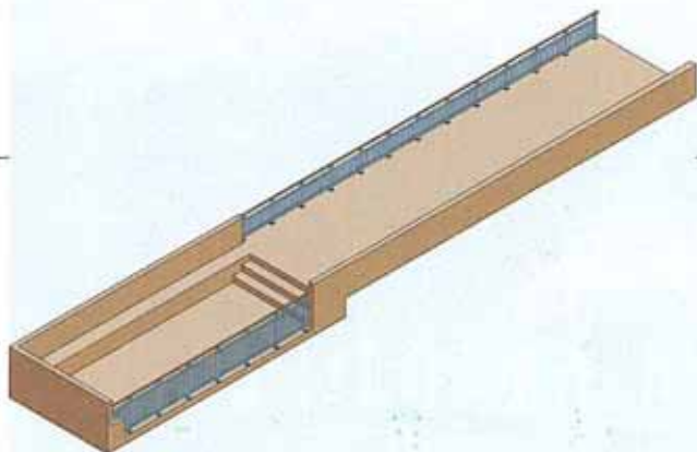
Isometrie uitkijkvlonder.
